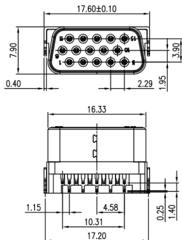
PN: G17DD1520308FHR PART NO. G17DD152 X 308FHR
